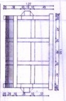
ELEVACIÓN FRONTAL ESTADO ACTUAL ESCALA 1:20
