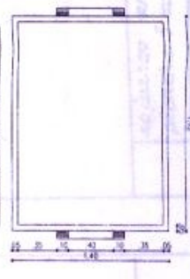
PLANTA ESTADO ACTUAL ESCALA 1:20
