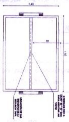
ADECUACIÓN DE TAPA VISTA INTERIOR ESCALA 1:20
