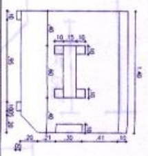
ELEVACIÓN LATERAL ESTADO ACTUAL ESCALA 1:20
