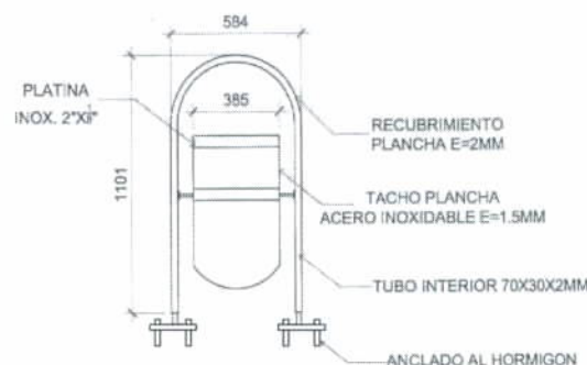
VISTA FRONTAL TACHO DE BASURA ESC 1:20
