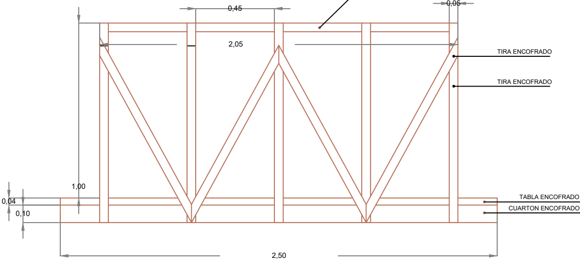
ELEVACION LATERAL Puentes PEATONALES DE MADERA PROV.:
