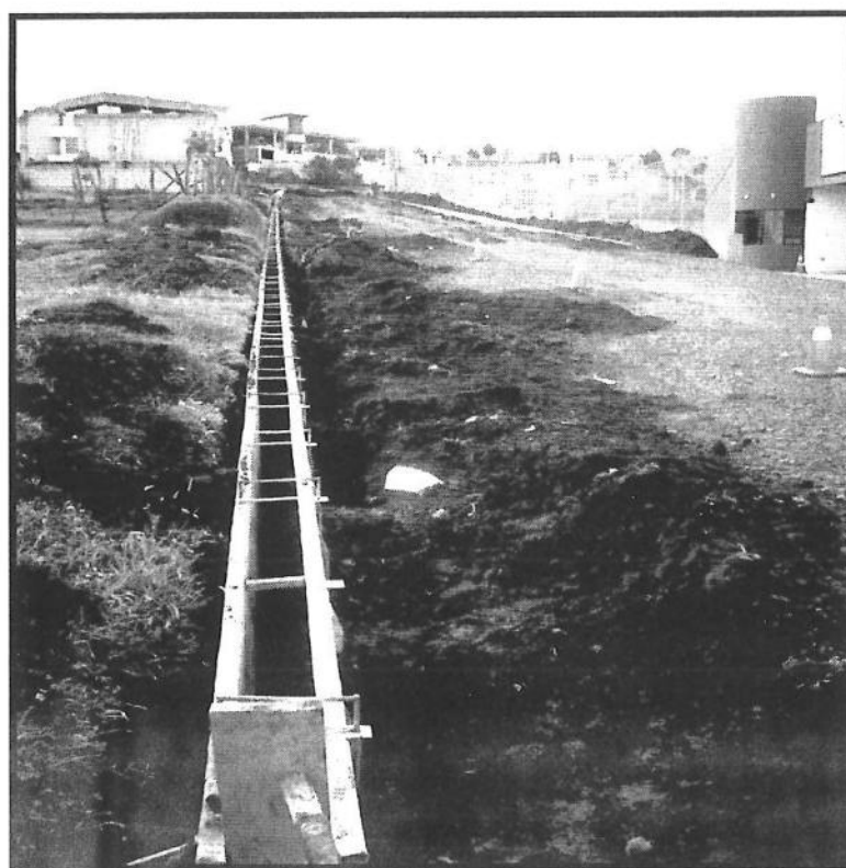
ENCOFRADO METALICO DE BORDILLO DE HORMIGON
